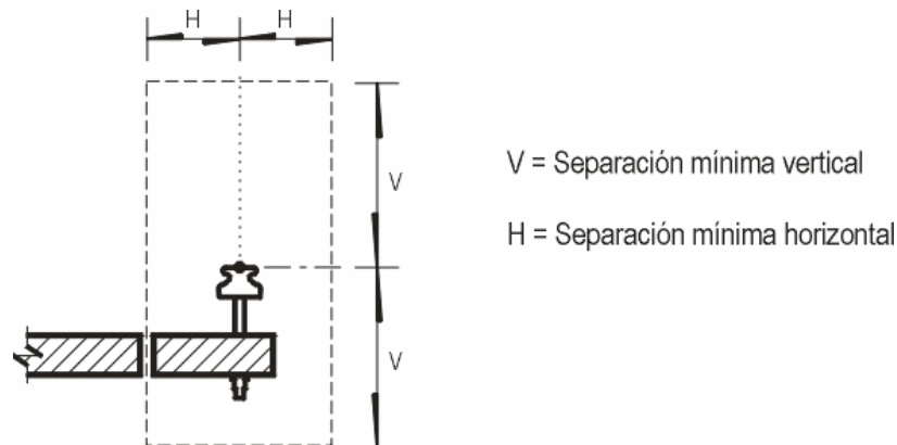
FIGURA.- 922-14
