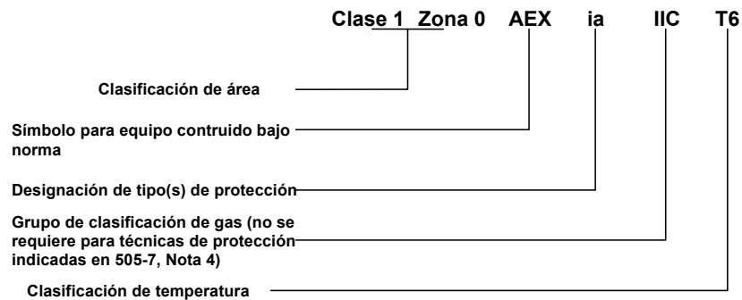
FIGURA 505-10 (b)(1)
